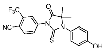
ABM-3
