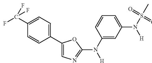
N-(3-((5-(4-(trifluoromethyl)phenyl)oxazol-2-yl)amino)phenyl)methanesulfonamide
