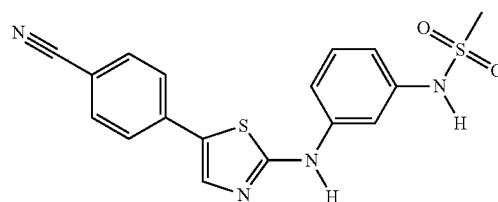
N-(3-((5-(4-cyanophenyl)thiazol-2-yl)amino)phenyl)methanesulfonamide
