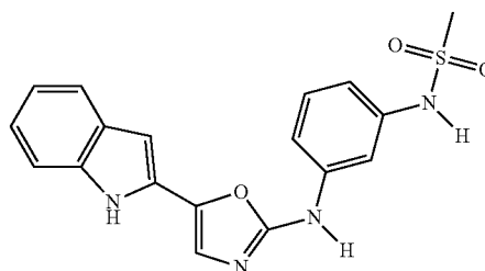
N-(3-((5-(1H-indol-2-yl)oxazol-2-yl)amino)phenyl)methanesulfonamide
