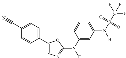
N-(3-((5-(4-cyanophenyl)oxazol-2-yl)amino)phenyl)-1,1,1-trifluoromethanesulfonamide
