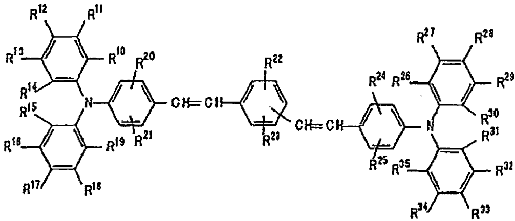
Allgemeine Formel (4)
