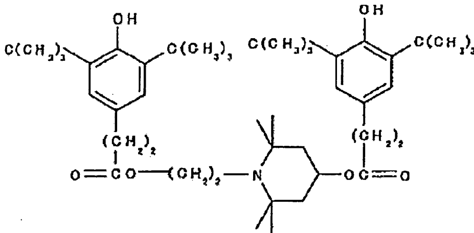
Strukturformel (3)
