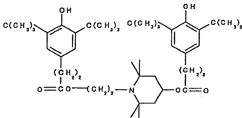
formule structurale (3)
