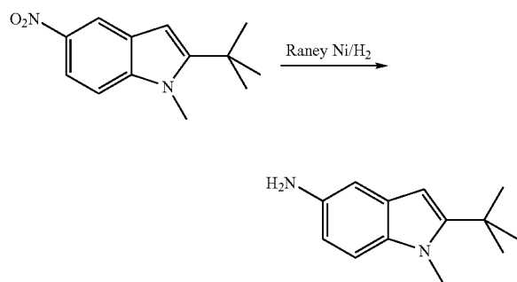
2-tert-Butyl-1-methyl-1H-indol-5-amine
