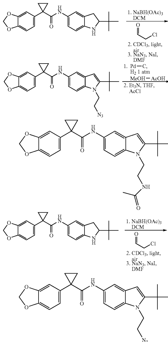
N-(1-(2-azidoethyl)-2-tert-butyl-1H-indol-5-yl)-1-(benzo[d][1,3]dioxol-5-yl)-cyclopropanecarboxamide
