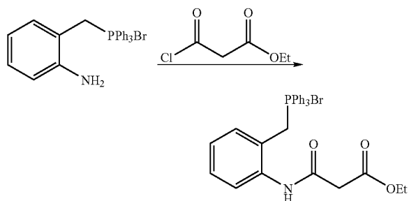
Triphenyl((ethyl(2-carbamoyl)acetate)-2-benzyl)phosphonium bromide
