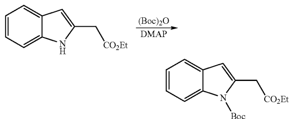
tert-Butyl 2-((ethoxycarbonyl)methyl)-1H-indole-1-carboxylate
