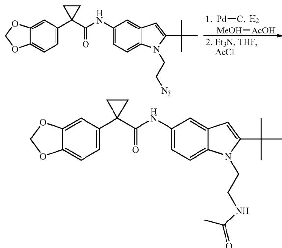
N-(1-(2-Acetamidoethyl)-2-tert-butyl-1H-indol-5-yl)-1-(benzo[d][1,3]-dioxol-5-yl)cyclopropanecarboxamide
