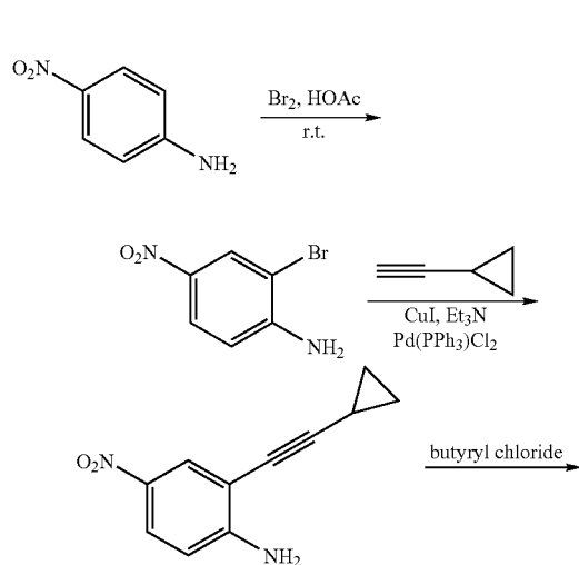
2-Cyclopropyl-1H-indol-5-amine
