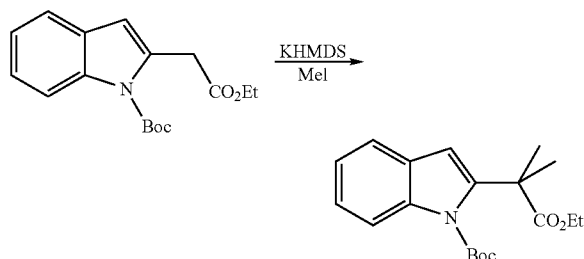
tert-Butyl 2-(2-(ethoxycarbonyl)propan-2-yl)-1H-indole-1-carboxylate
