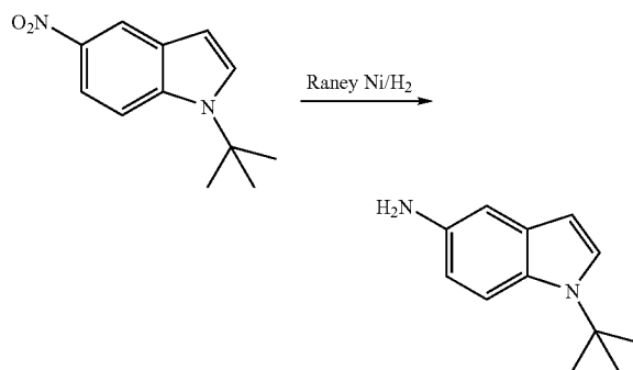
1-tert-Butyl-1H-indol-5-amine
