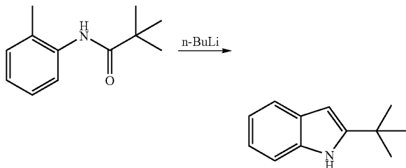
2-tert-Butyl-1H-indole
