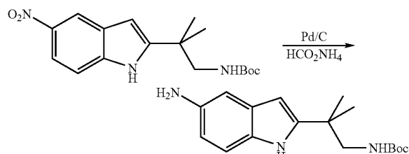
tert-Butyl 2-(5-amino-1H-indol-2-yl)-2-methylpropylcarbamate
