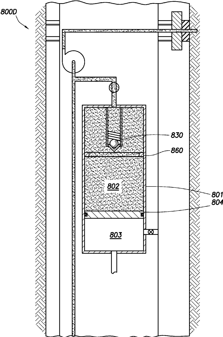
FIG. 7D
