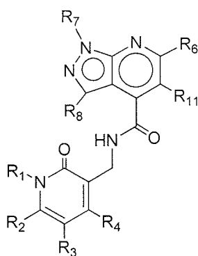
(IIa)
