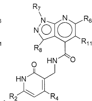
(IIId)
