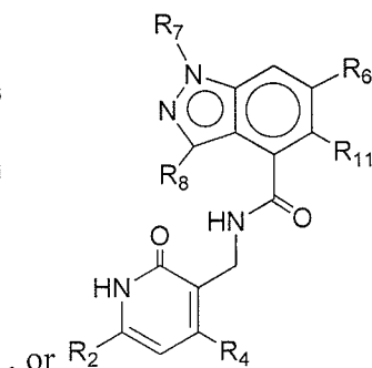
(IIId)
