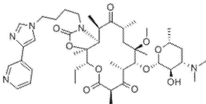
Telithromycin
