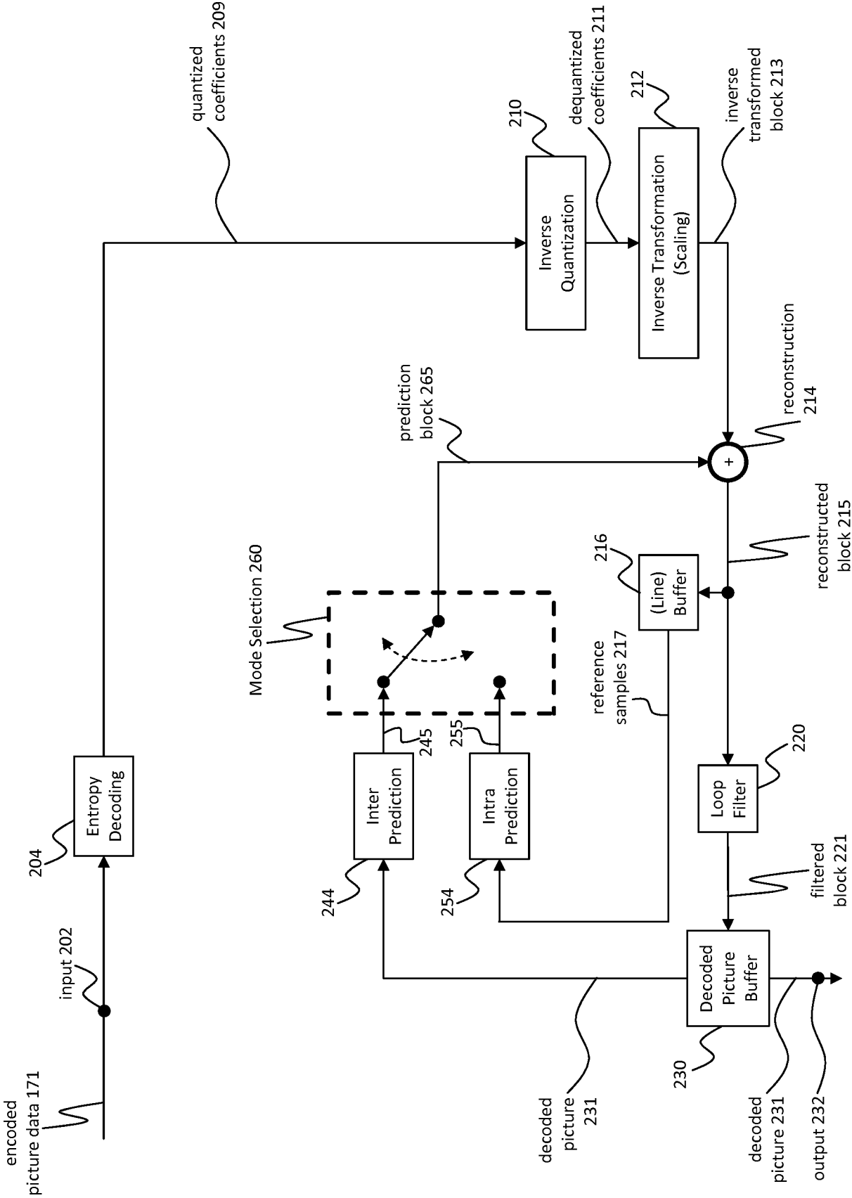
Decoder 200 Fig. 2
