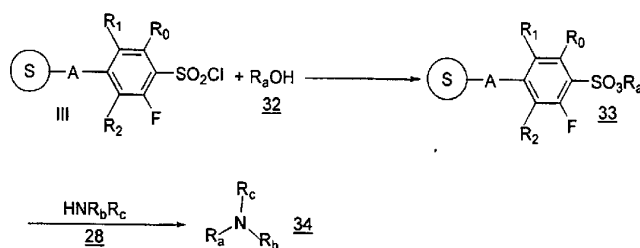
Scheme 9a
