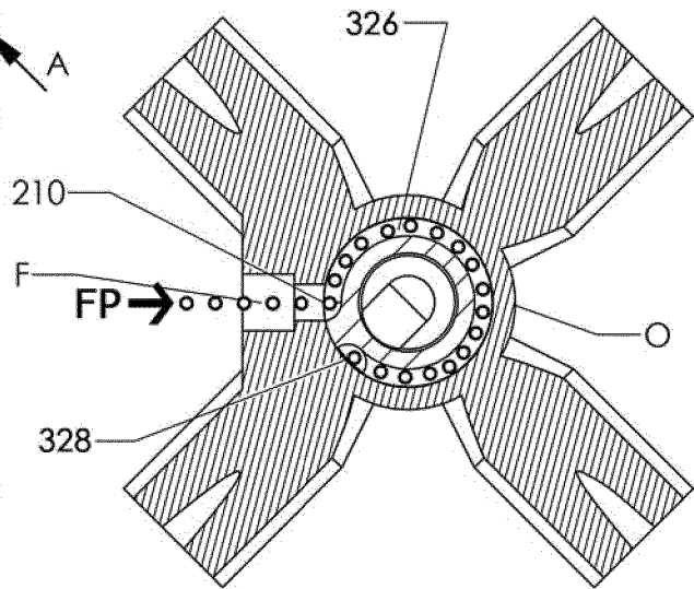
SECTION B-B FIG. 7D
