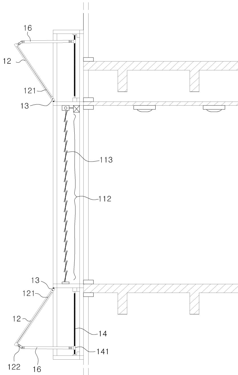
도면4
