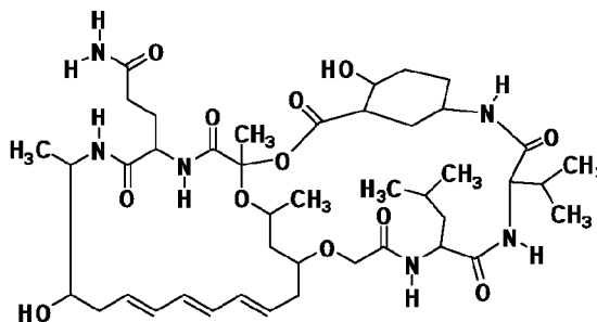
Chromamide A (1)
