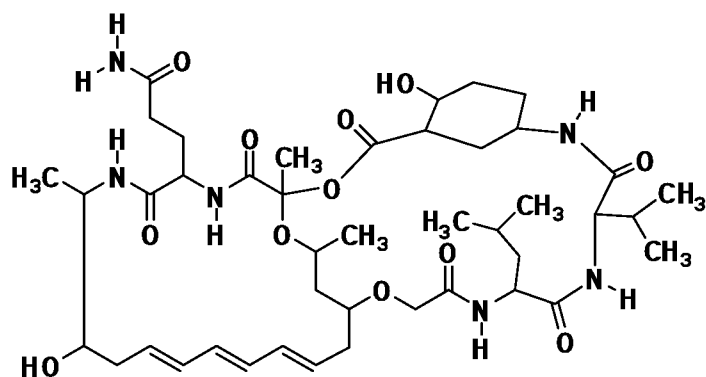
Chromamide A (1)
