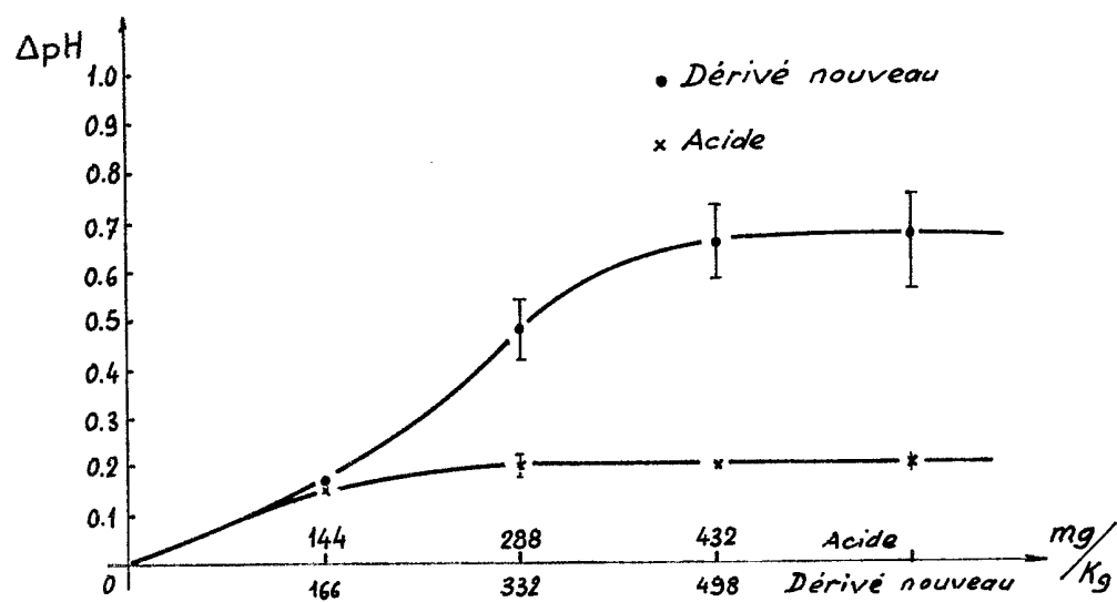
Graphique 1 - Représentation graphique des \Delta pH en fonction des doses du dérivé nouveau et de l'acide 2-(4-isobutylphényl)propionique.
