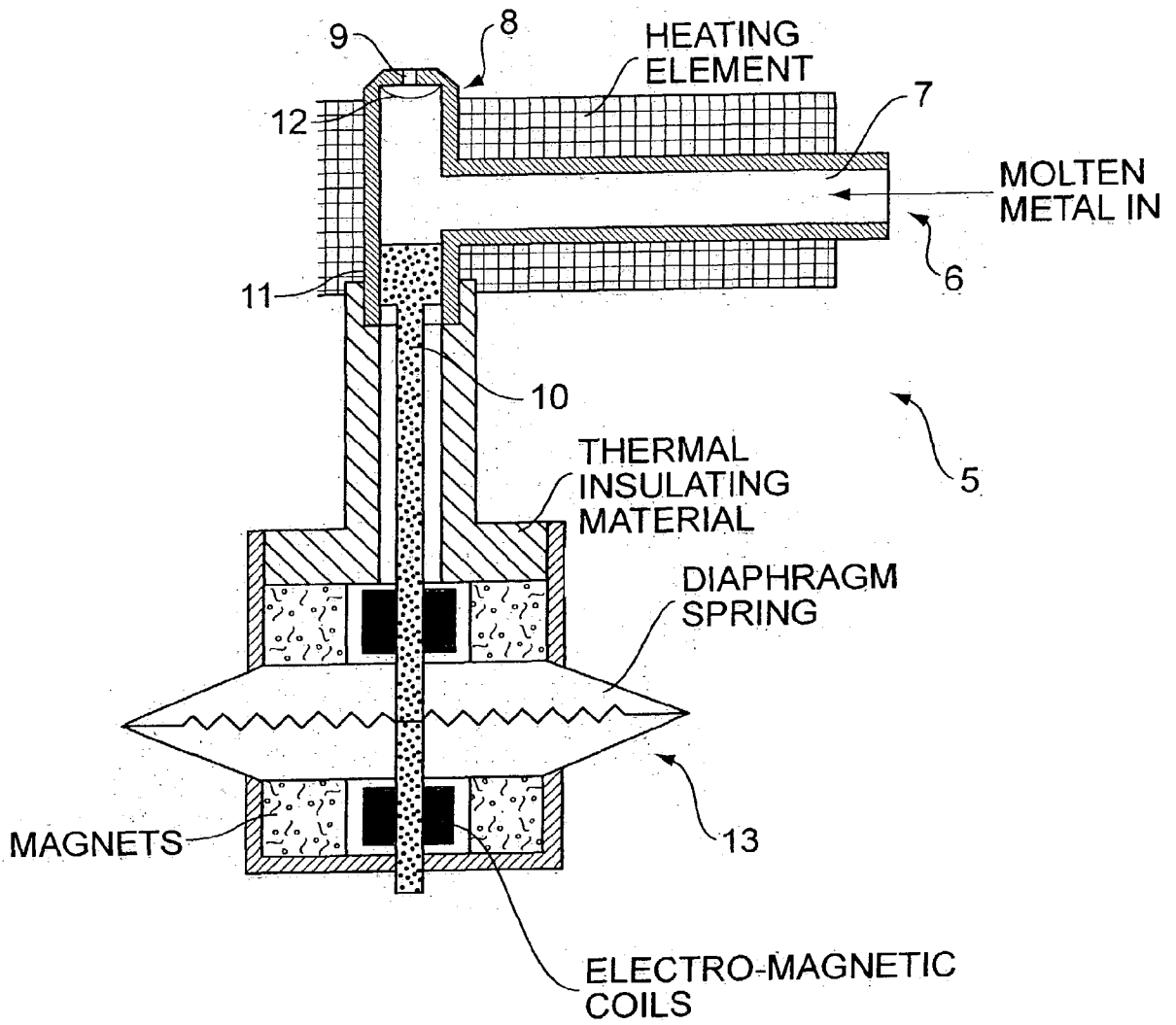
FIG. 2A
