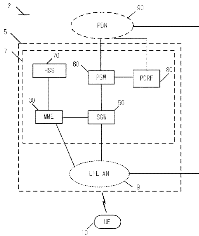
FIG. 16A
