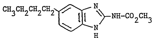
Parbendazole
