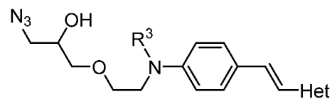
Compounds E1
