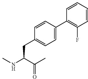
Bip(2'-F)
