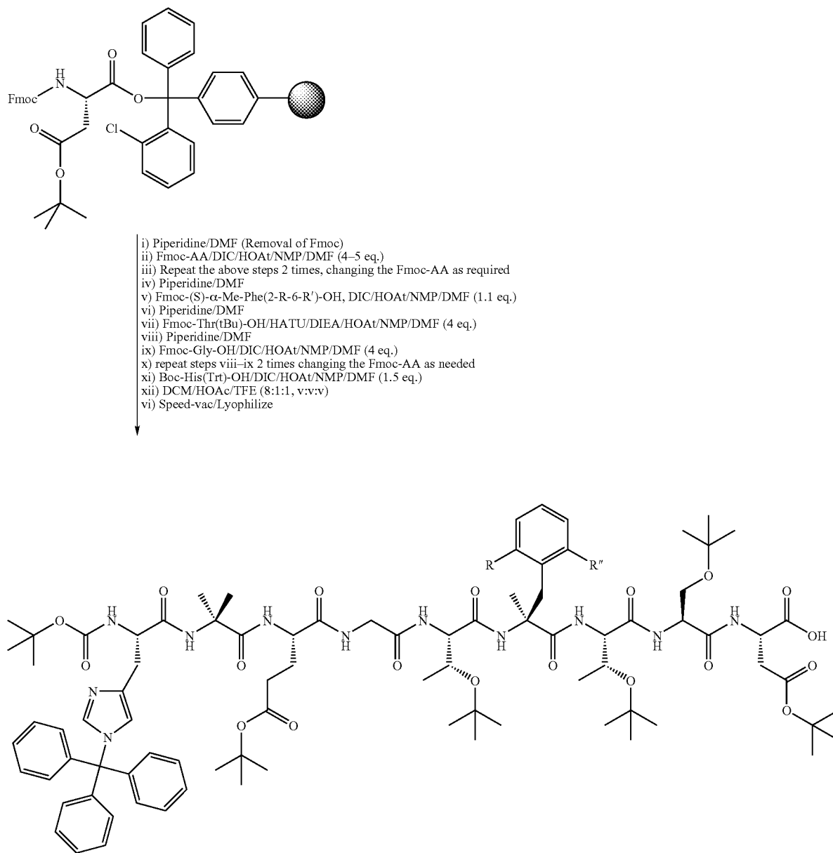
SCHEME 9A
