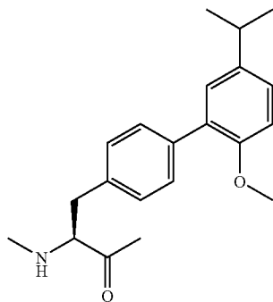
Bip(2'-MeO-5'-isopropyl)
