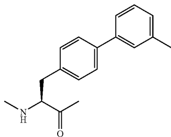
Bip(3',5'-di-Me)
