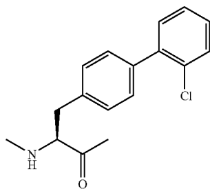
Bip(2'-Cl)
