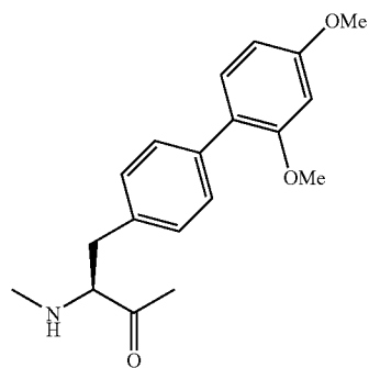
Bip(2',4'-di-OMe)
