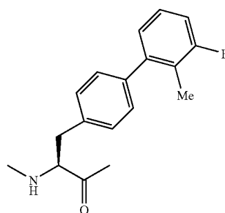
Bip(2'-Me-3'-F)
