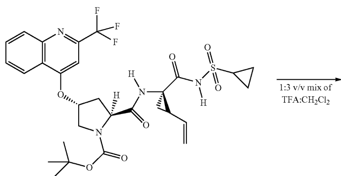
Example 180d
