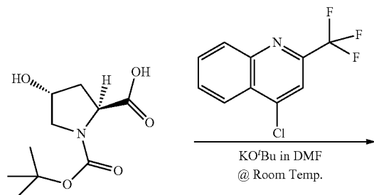
Example 180a
