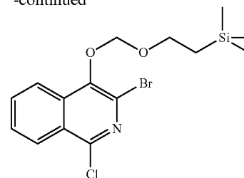
Example 222
