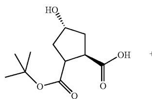
Example 180a
