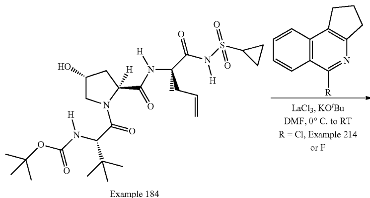
Example 184
