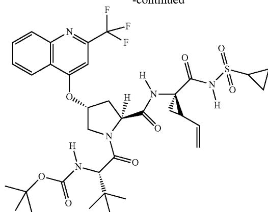
Example 180
