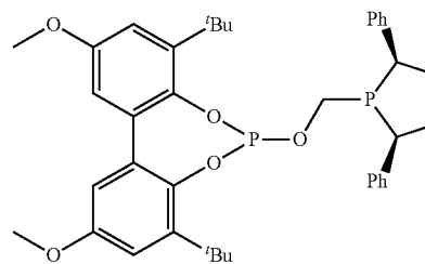
(tropos,meso)-2
