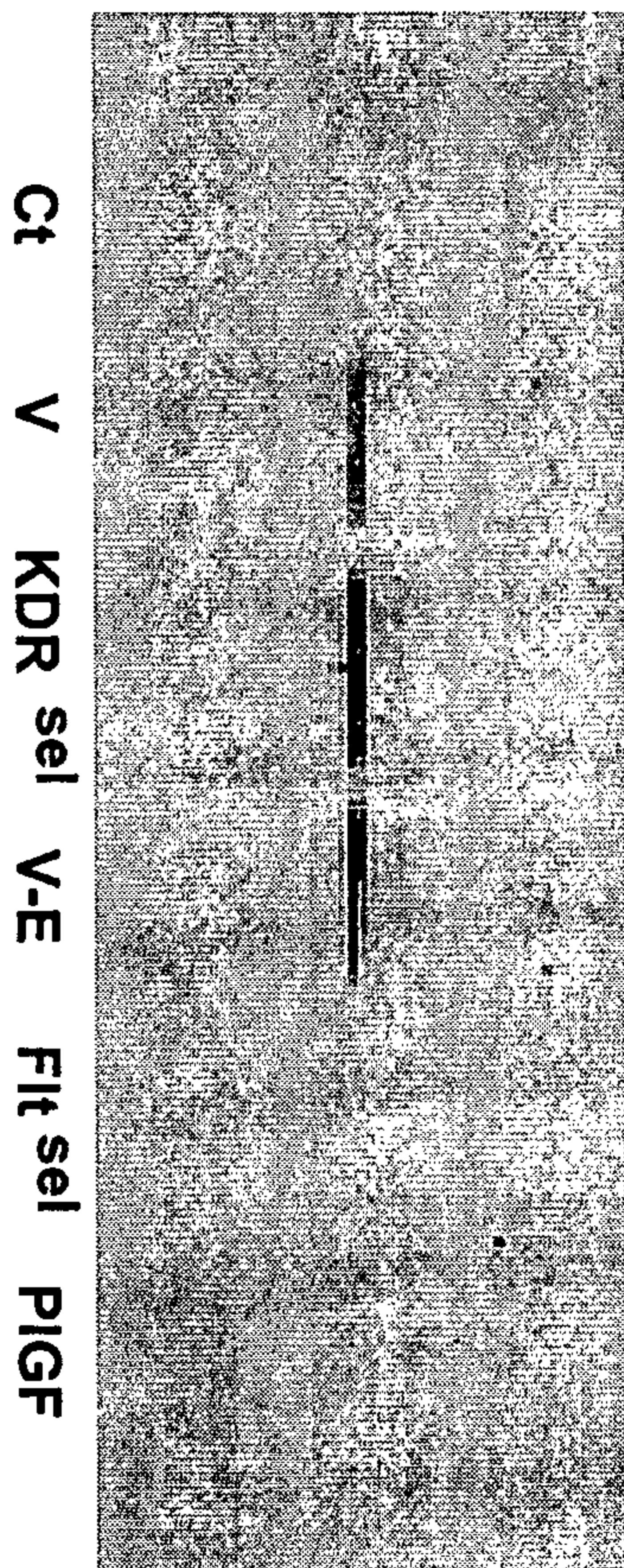
pPERK1/2
