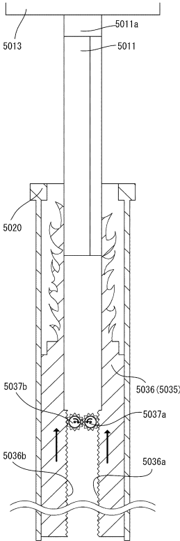
(A) オーラ部材 5 0 3 5 の完全収容状態
