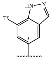
1H-Benzotriazol-5-yl
