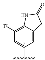
3H-Benzoxazol-2-on-6-yl
