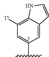
1H-Indol-5-yl
