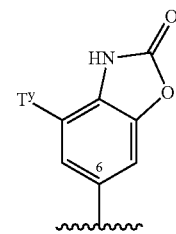
1,3 Dihydro-benzoimidazol-2-on-5-yl
