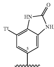
1,3 Dihydro-benzoimidazol-2-on-5-yl
