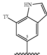
1H-Indazol-5-yl
