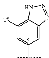
1H-Benzotriazol-5-yl
