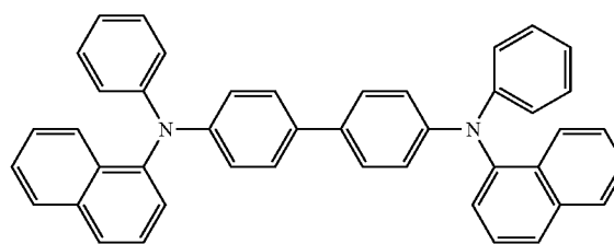
\alpha -NPD
