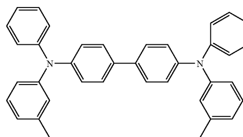
TPD
