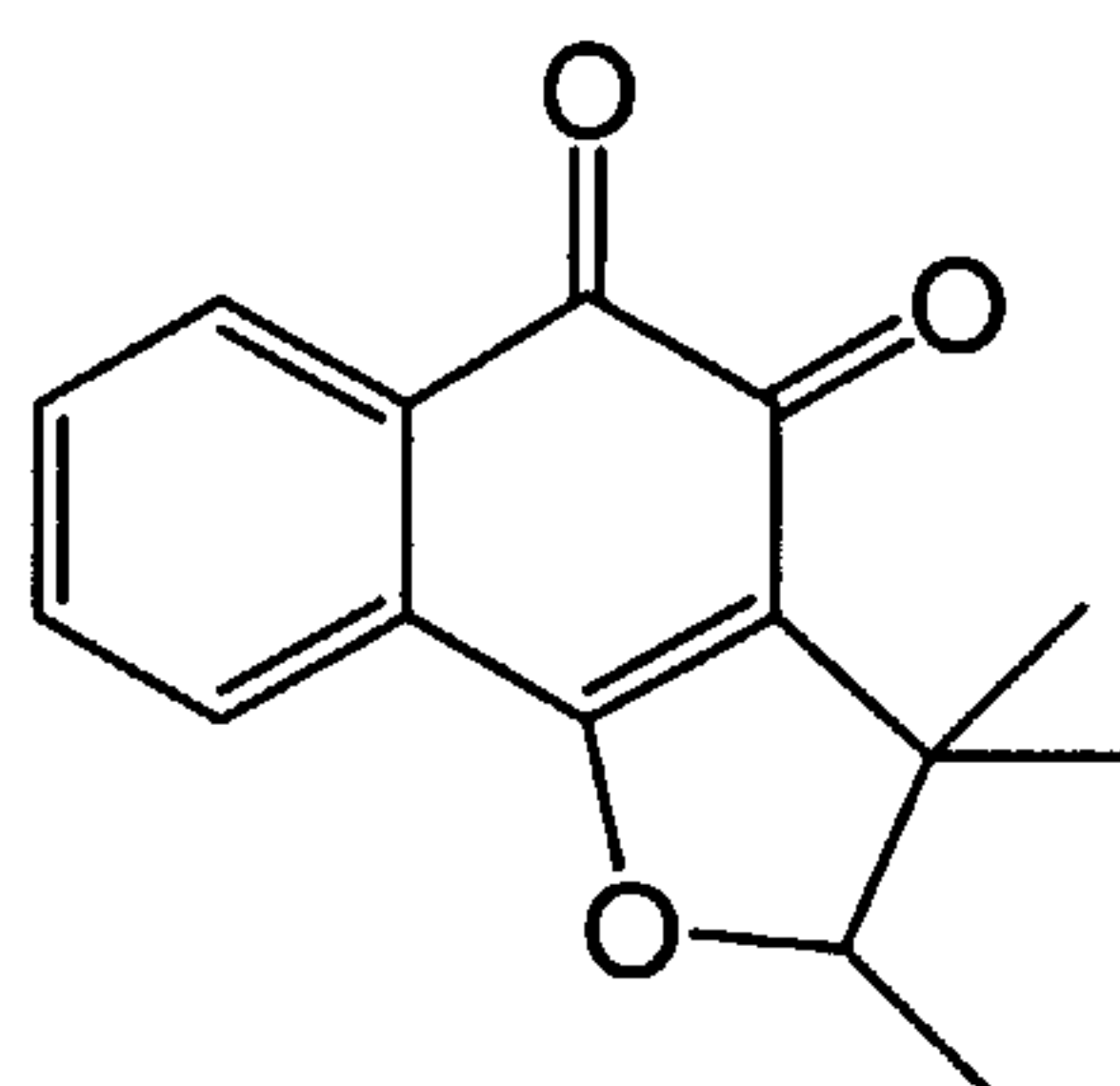
Dunnione
