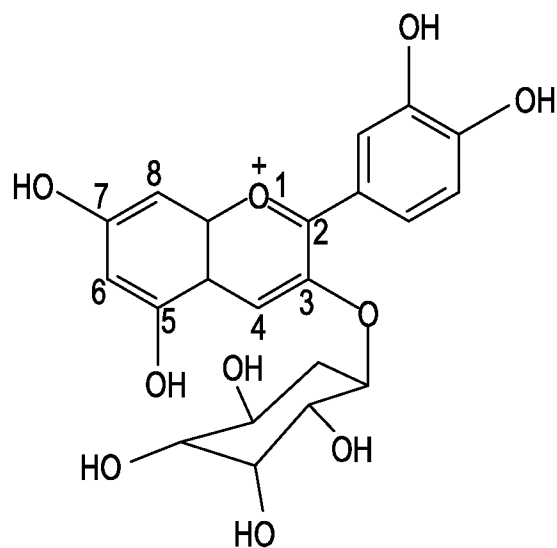
I: CYANIDIN -3- GLUCOSIDE
