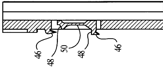
FIG. 3D B-B
