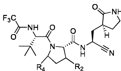
(VIII-1)
