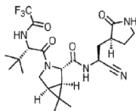
PF-07321332
