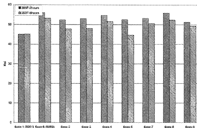
Example 1 Alloys - Tensile Yield Strength (ksi)
