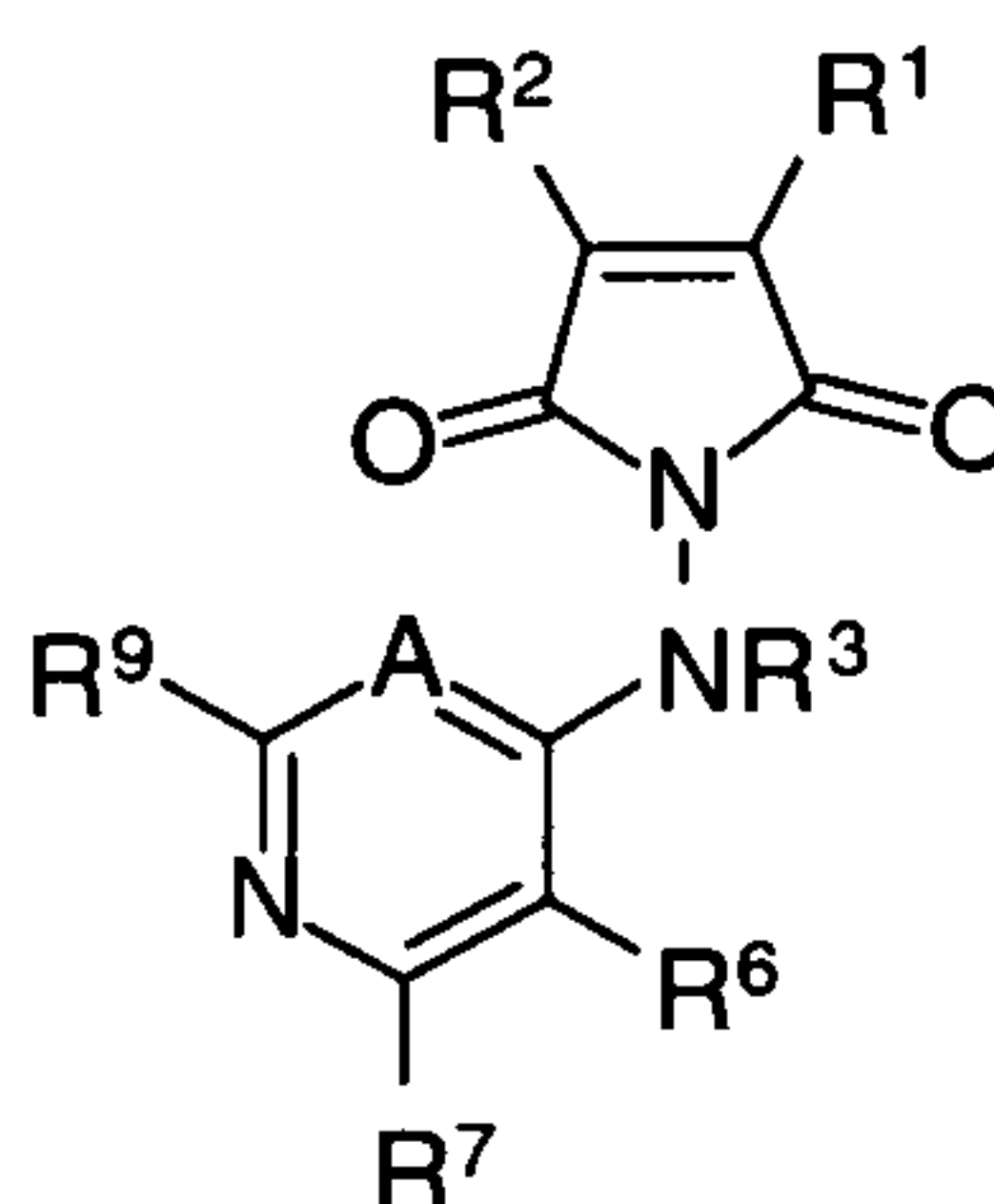
( XI )
