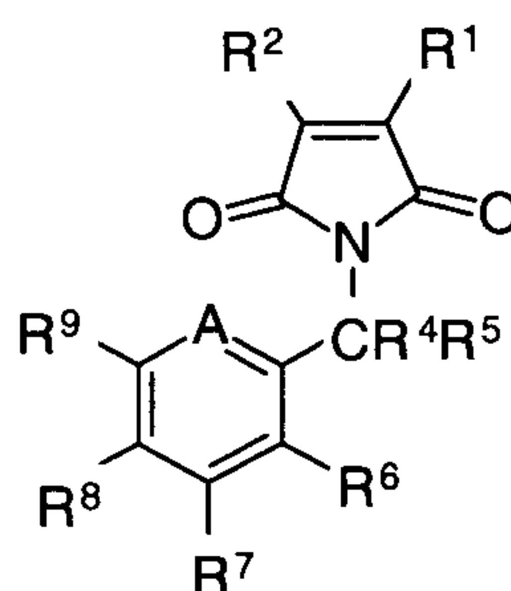
( VI )
