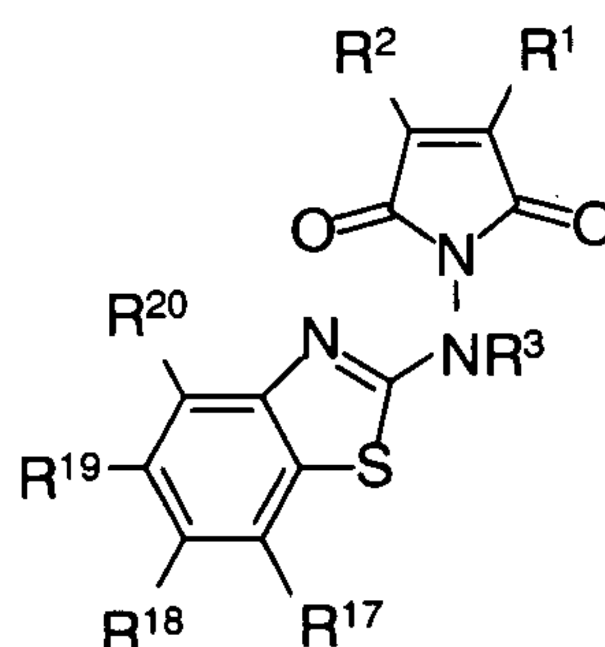
( VII )
