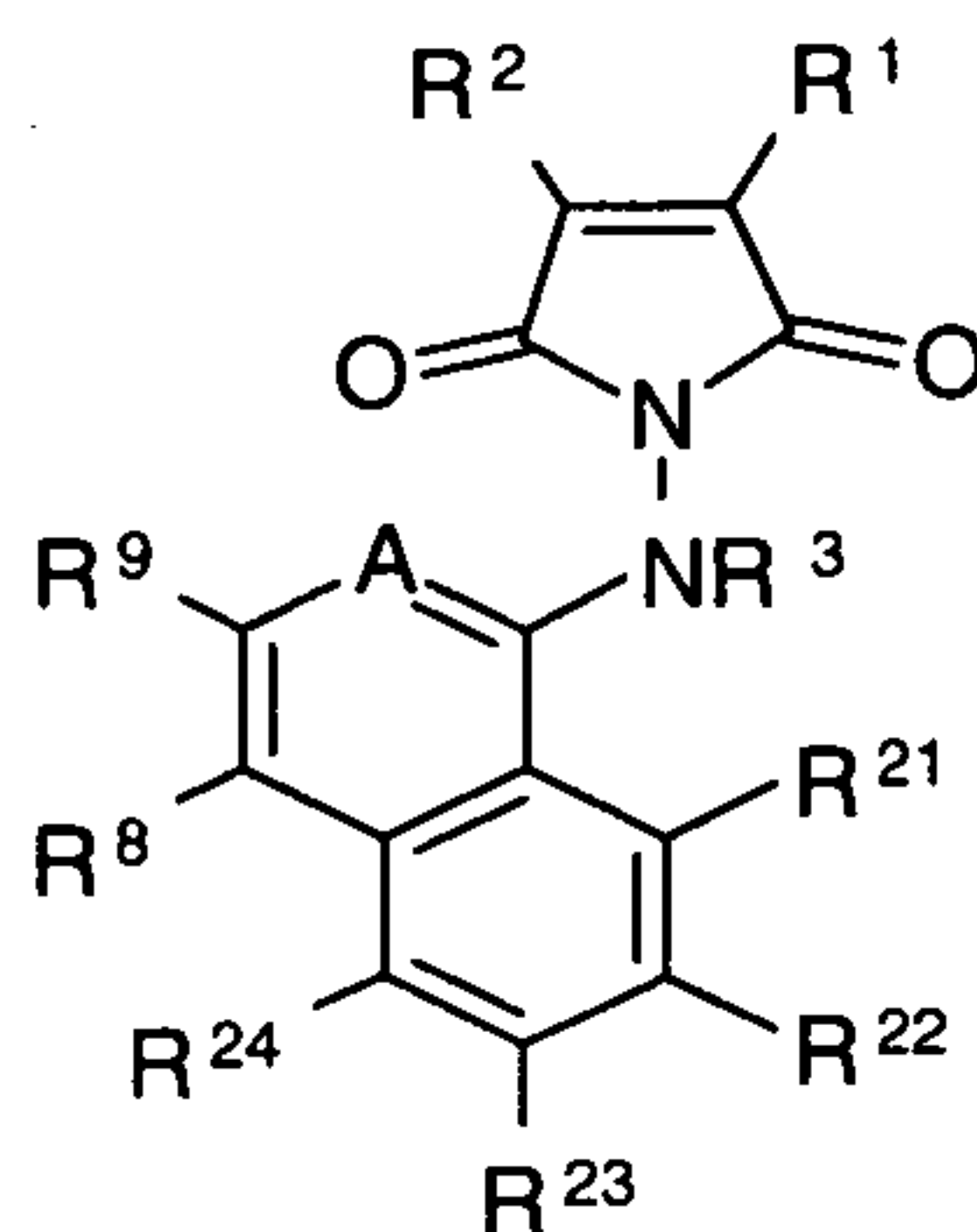
( VIII )
