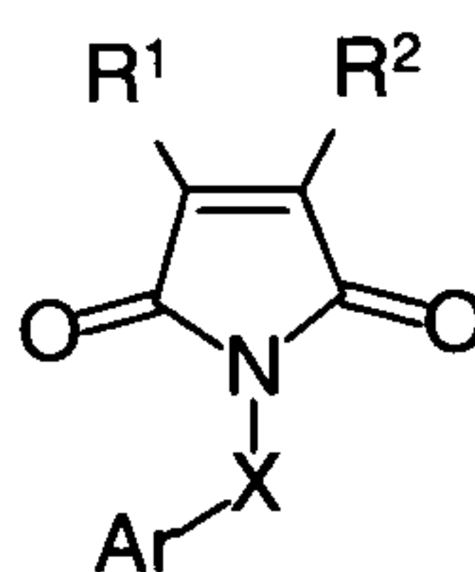
( I )
