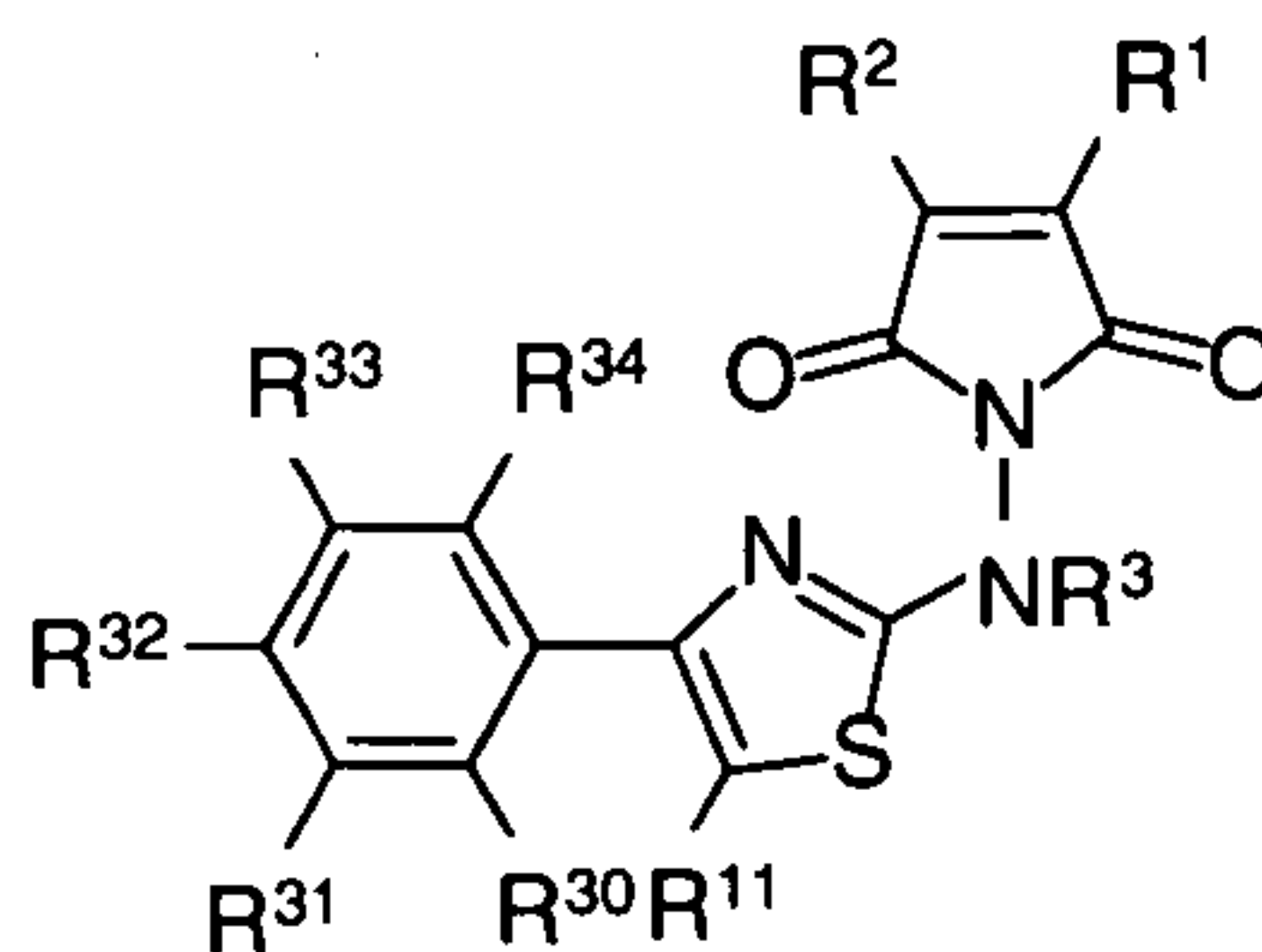
( X )
