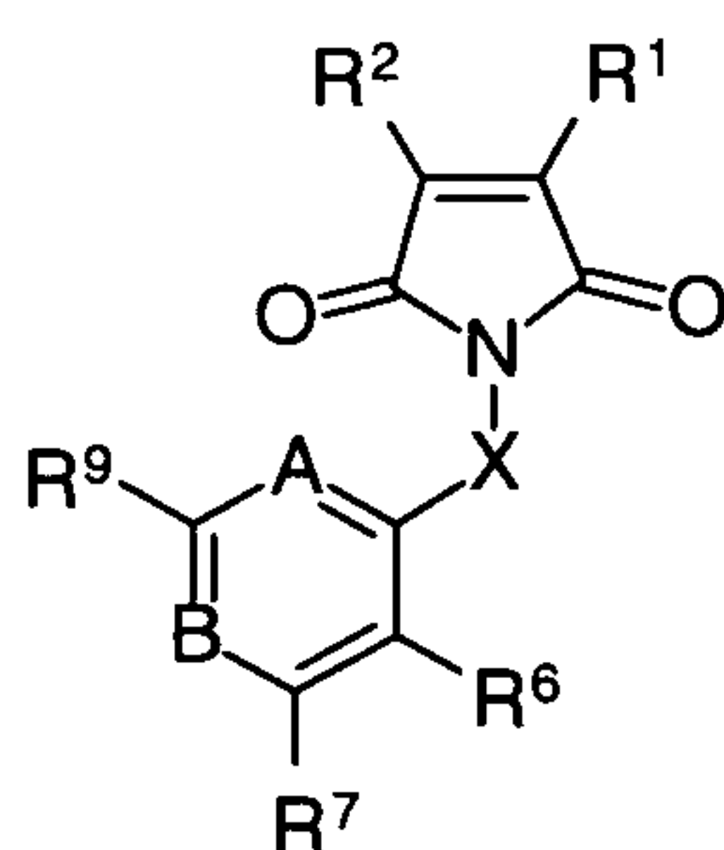
( II )
