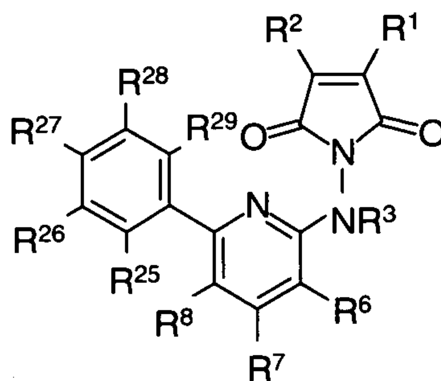
( IX )
