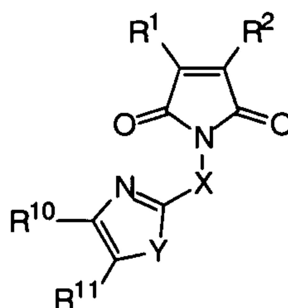
( III )
