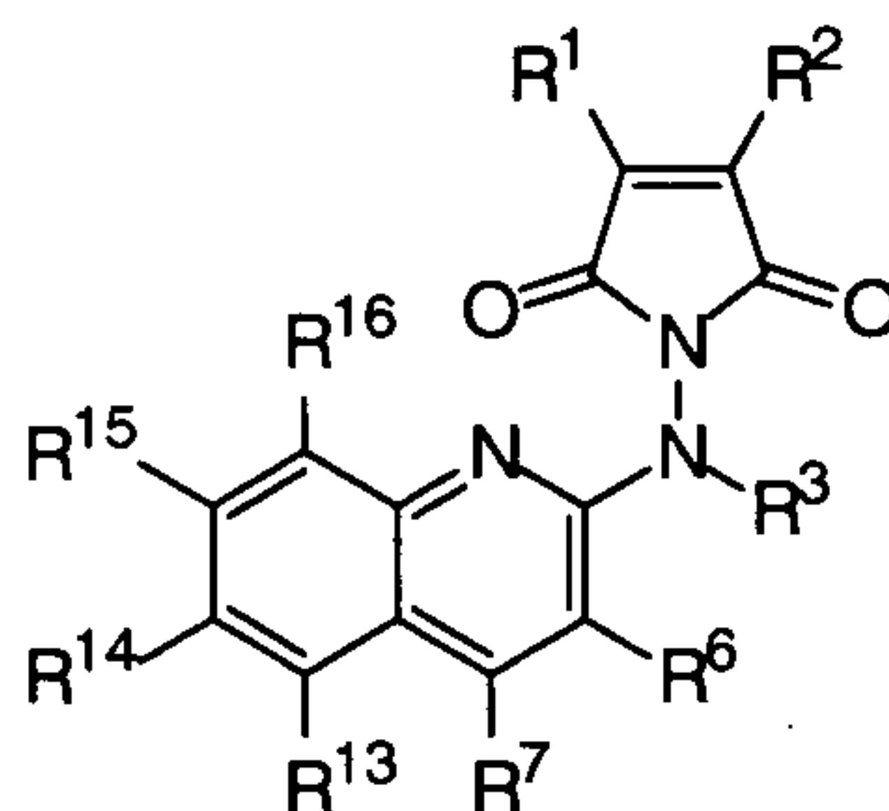
( V )
