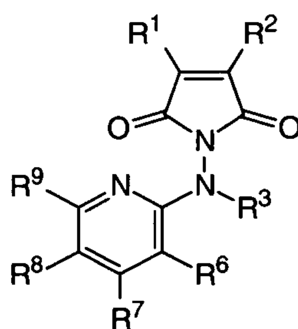
( IV )
