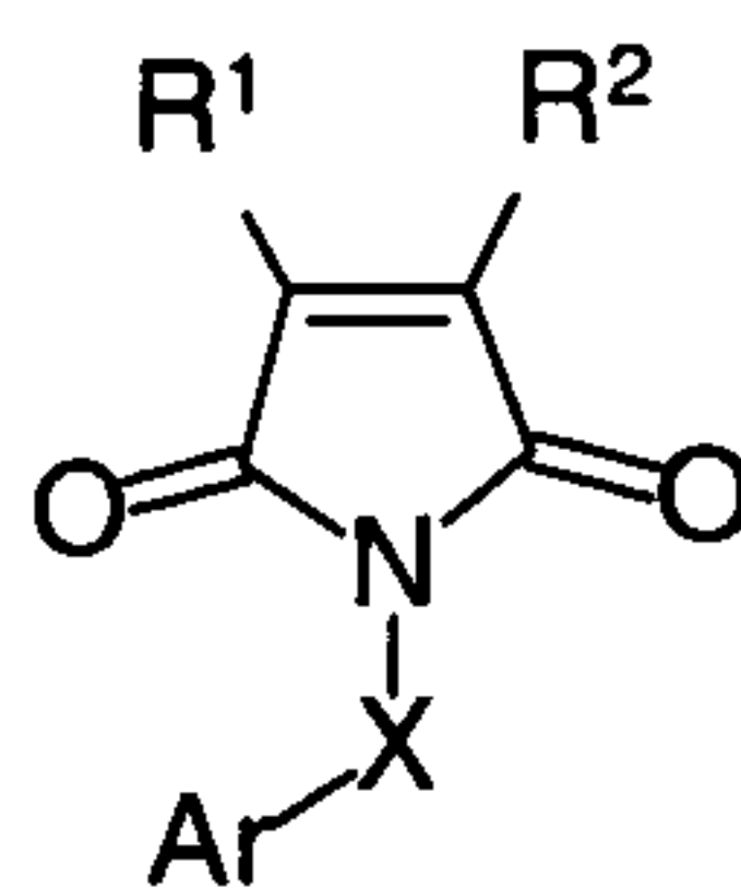
( I )
