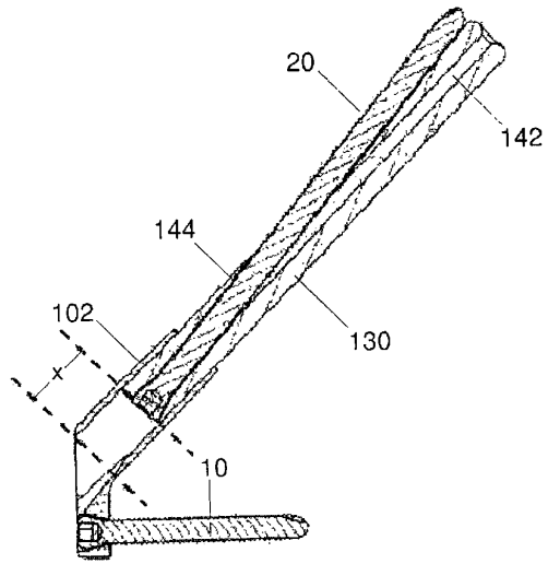
도면23
