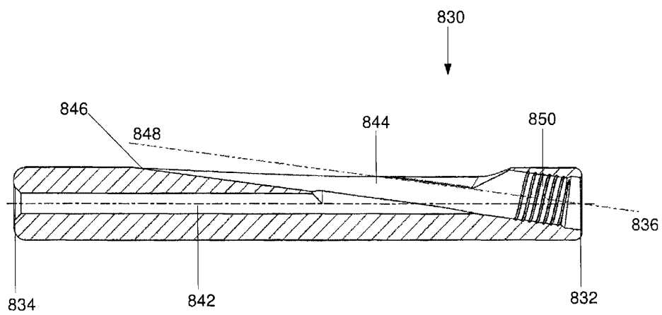
도면43
