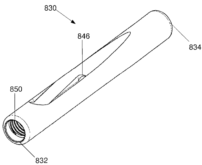
도면43
