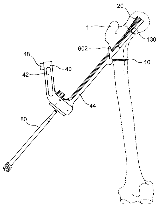
도면32
