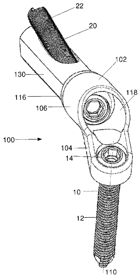
도면3
