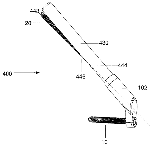
도면30
