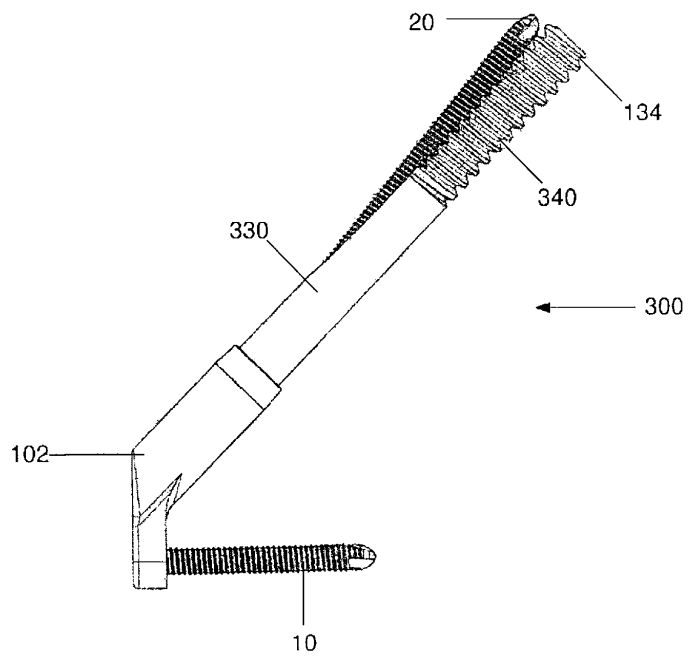
도면28
