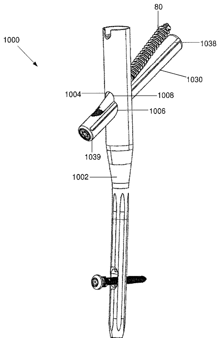
도면53
