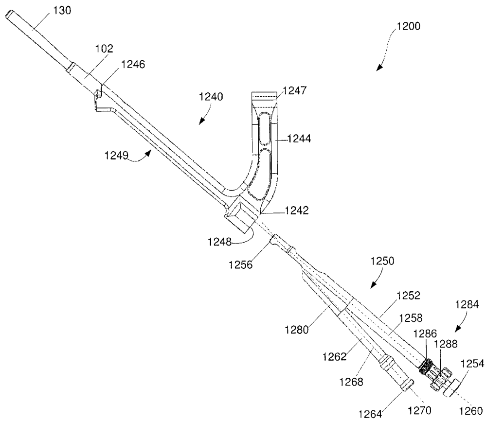
도면58
