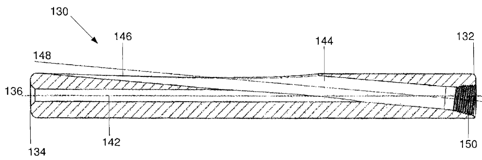
도면9
