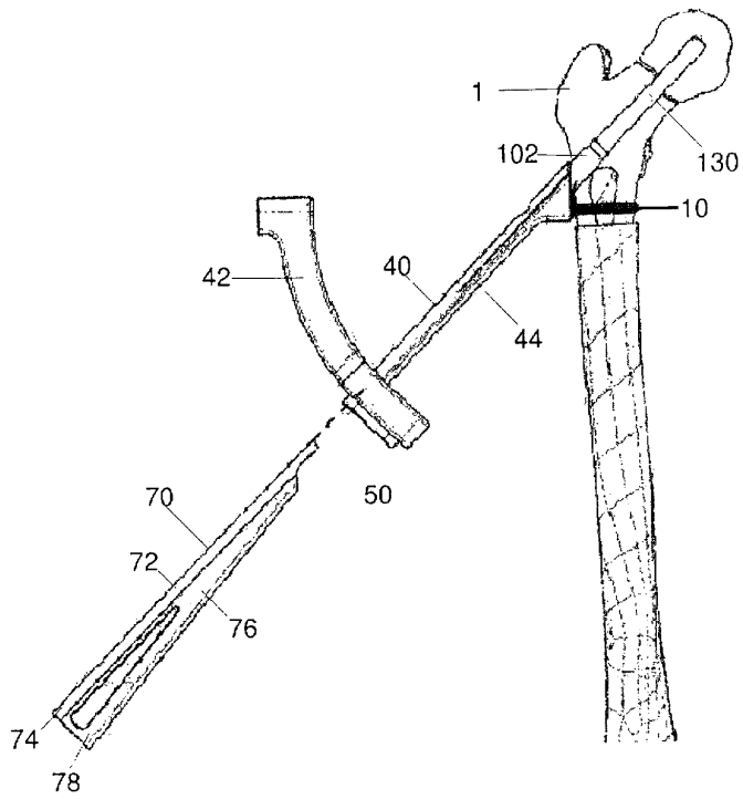
도면17
