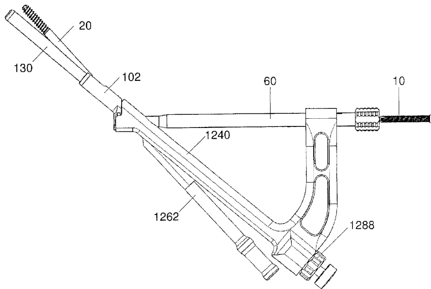
도면62
