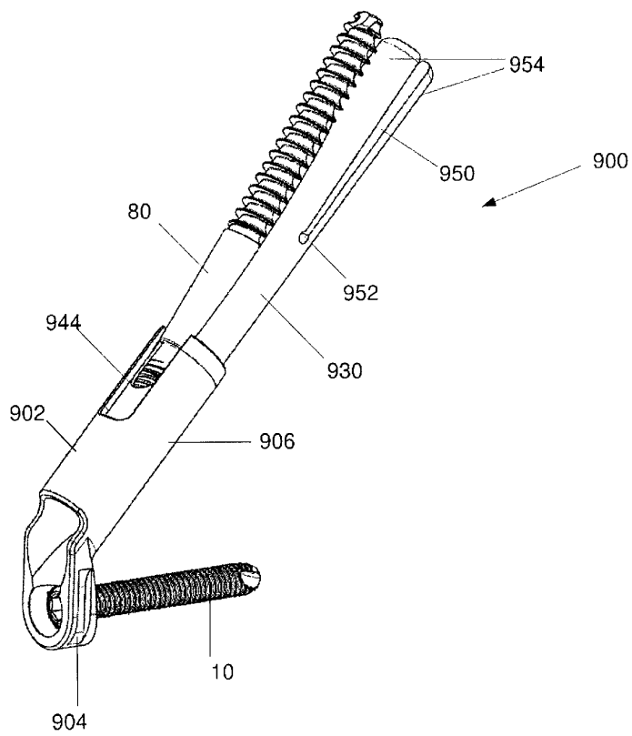
도면51
