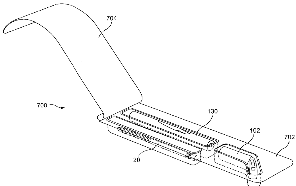
도면34
