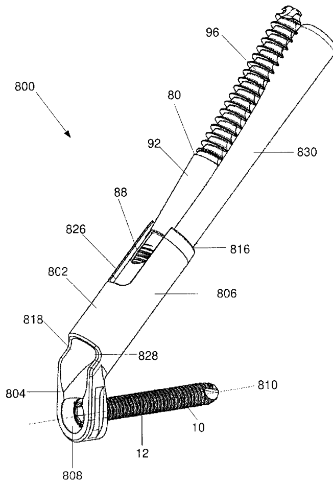
도면37
