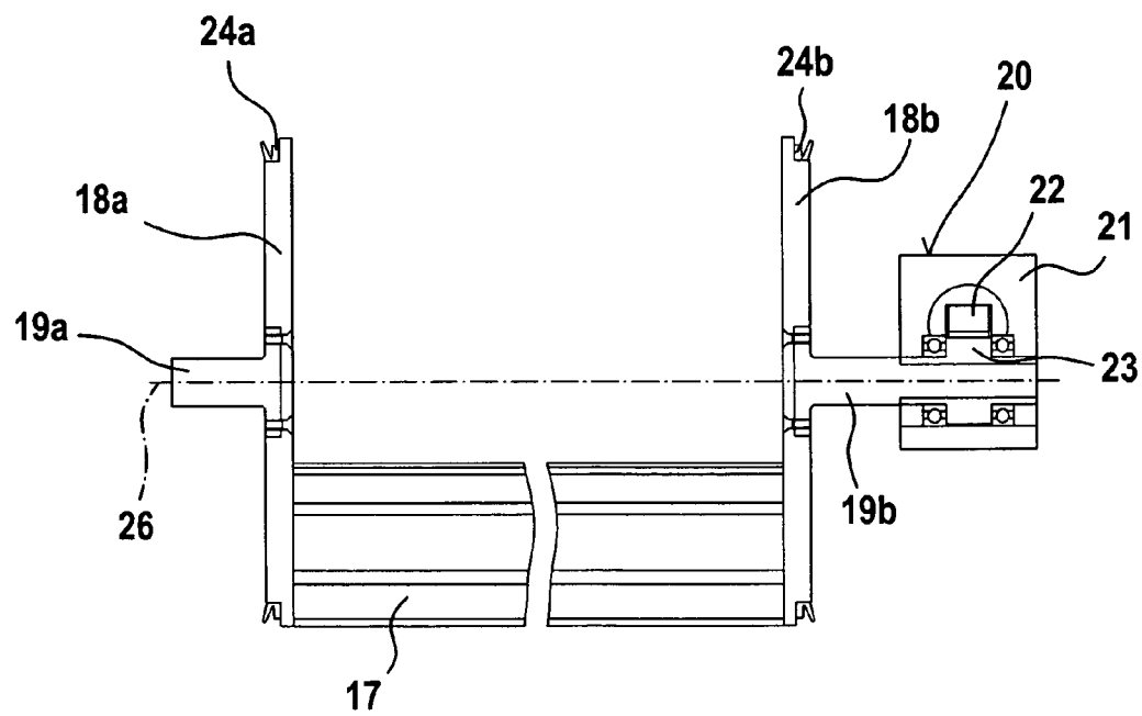
Fig. 3b I-I
