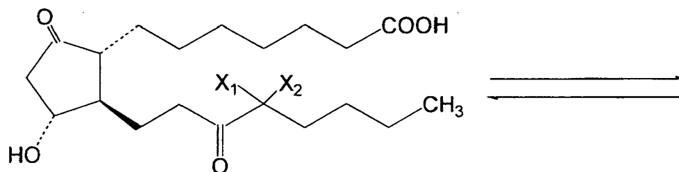
Tautomer I
