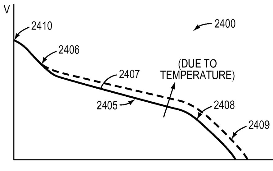
FIG. 24 V - I CURVE
