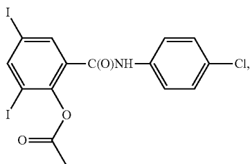
clioxanide
