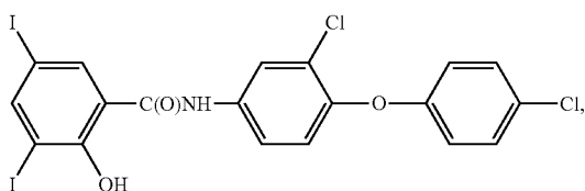
rafoxanide
