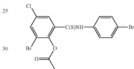
brotitanide
