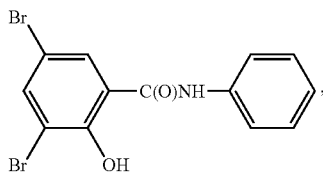
dibromosalalan
