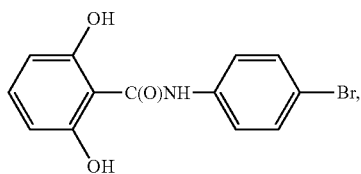
resorantel
