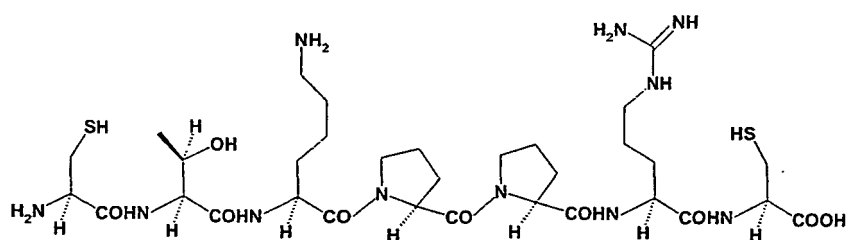
H-Cys-Thr-Lys-Pro-Pro-Arg-Cys-OH
