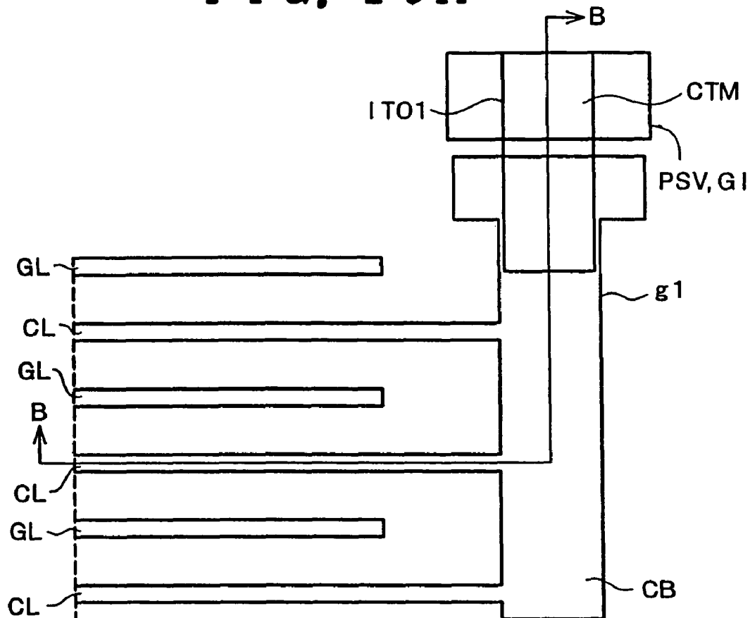
FIG. 10B
