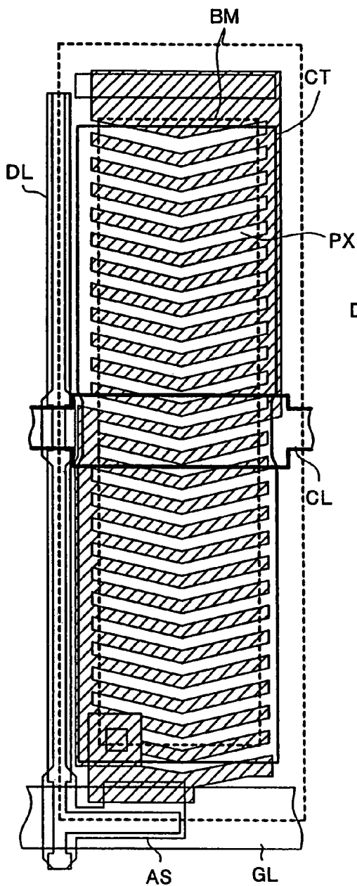
FIG. 18A
