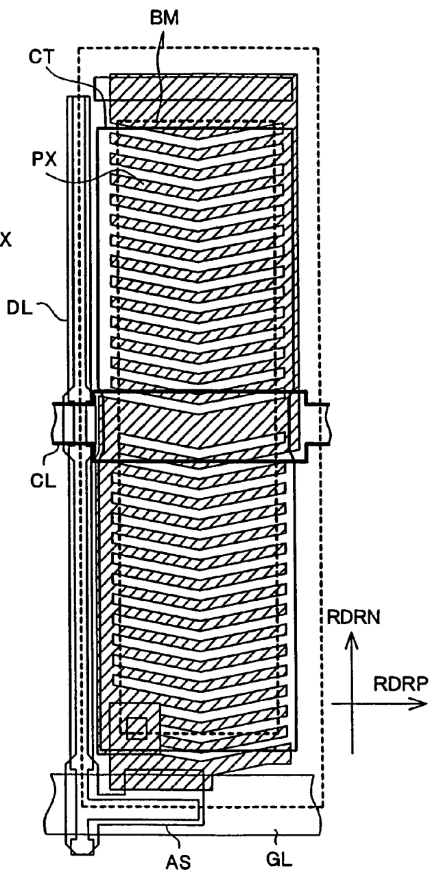
FIG. 18B
