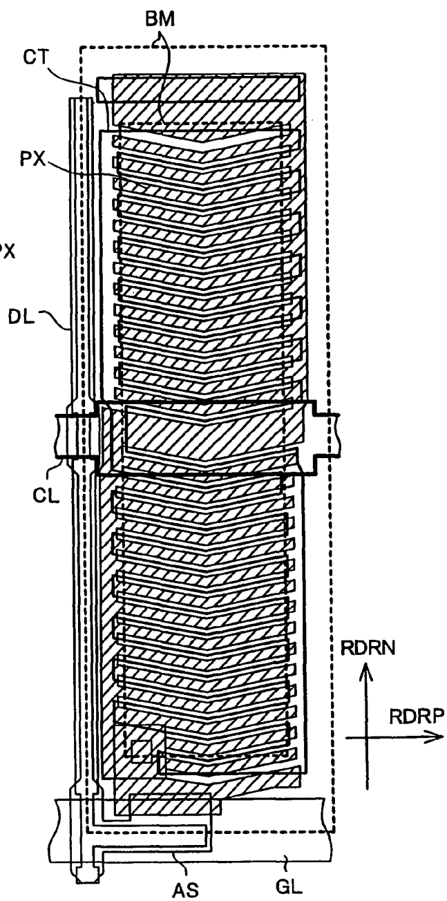
FIG. 19B
