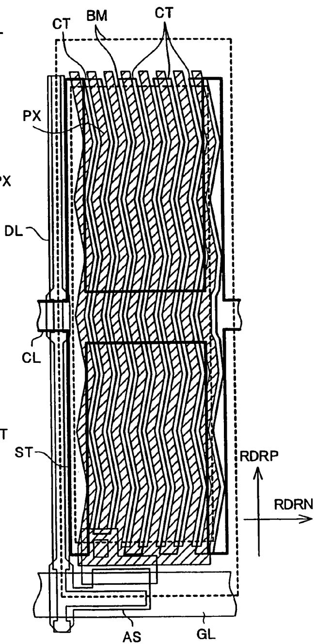
FIG. 17B
