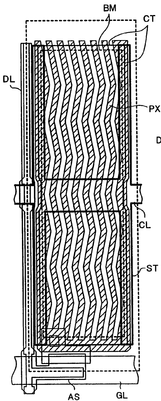
FIG. 17A
