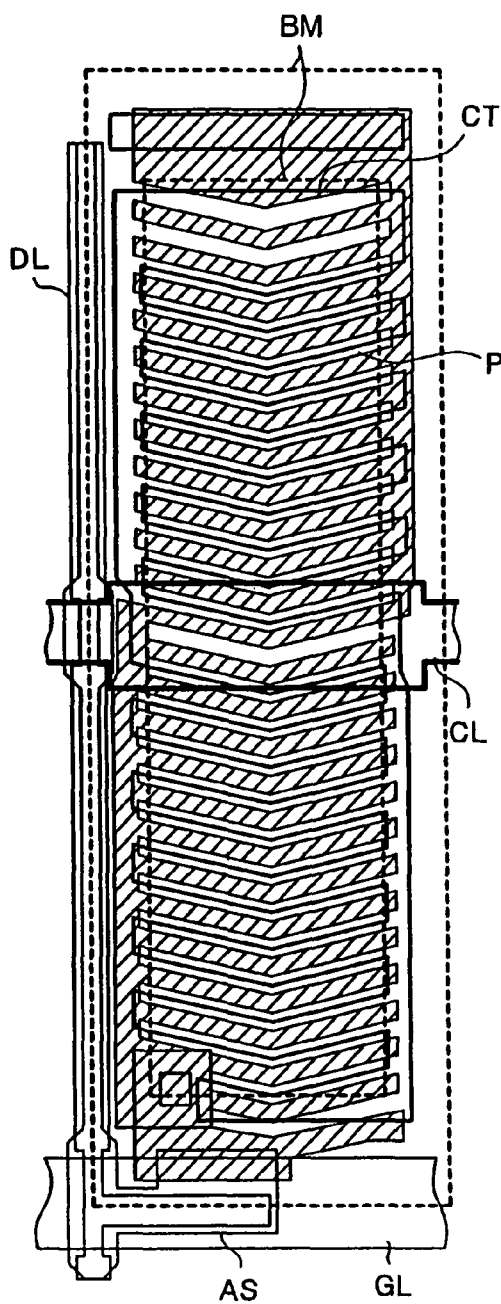
FIG. 19A
