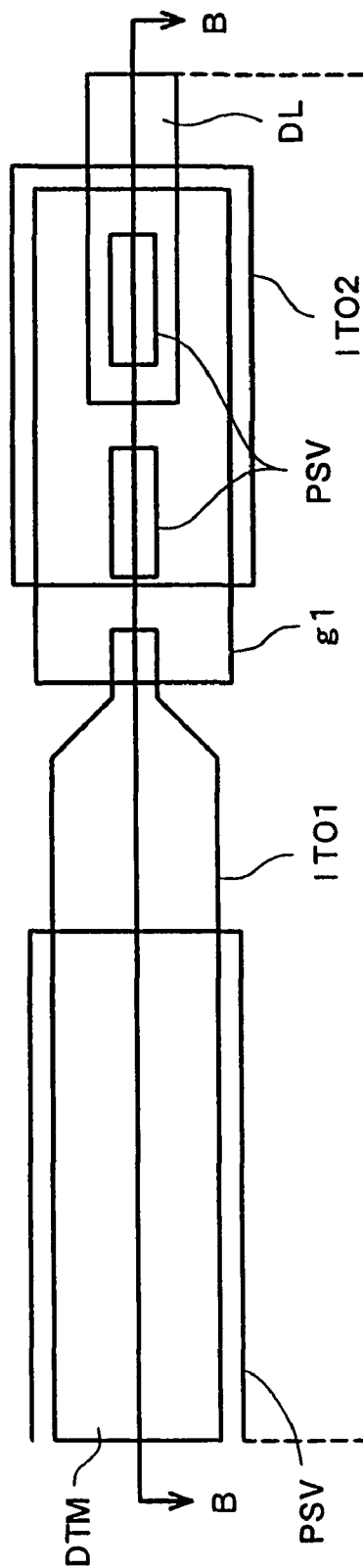
FIG. 9A
