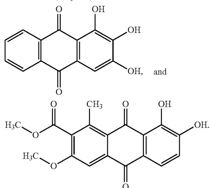
(Purpurin)
