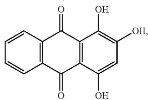
(Purpurin)
