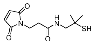
MPBT: maleimidoPropionamidoButylThio
