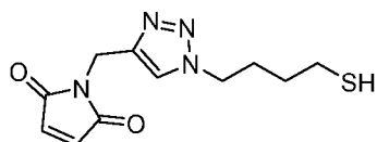
MaleimidoMethylTriazoleButaneThiol (MMTBT)
