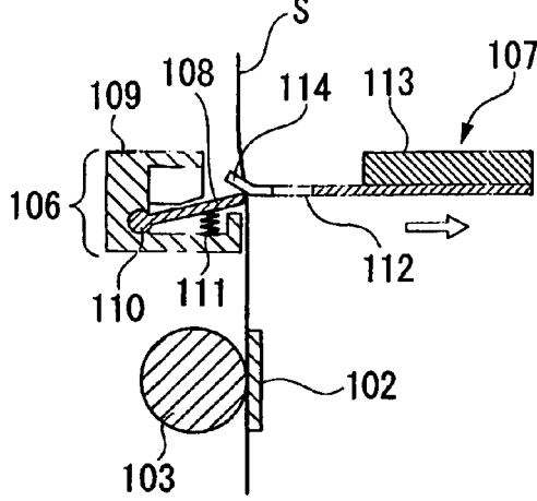
FIG. 7D PRIOR ART
