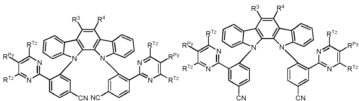
Formula Va
