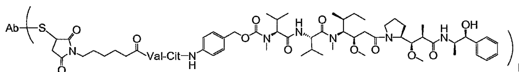
Ab-MC-vc-PAB-MMAE
