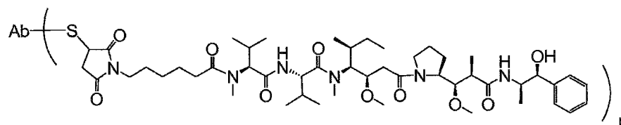
Ab-MC-MMAE
