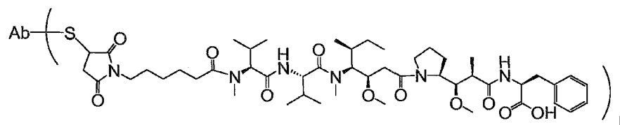
Ab-MC-MMAF
