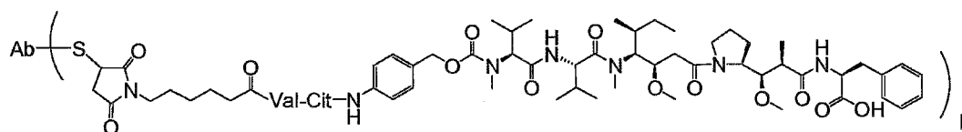
Ab-MC-vc-PAB-MMAF
