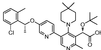
Example 282
