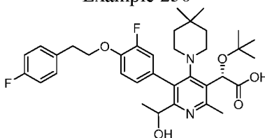
Example 236
