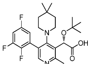
Example 174
