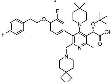
Example 231
