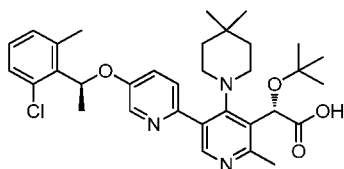
Example 281
