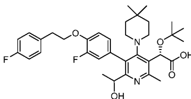
Example 237
