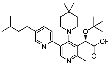
Example 273
