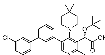
Example 144
