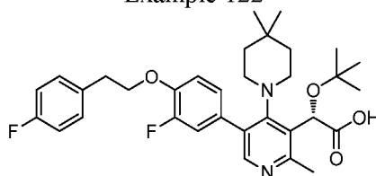
Example 122
