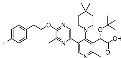
Example 448
