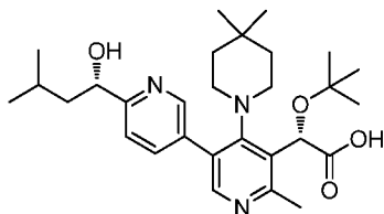
Example 432
