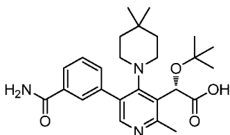
Example 146
