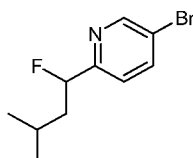
5-Bromo-2-(1-fluoro-3-methylbutyl) pyridine:
