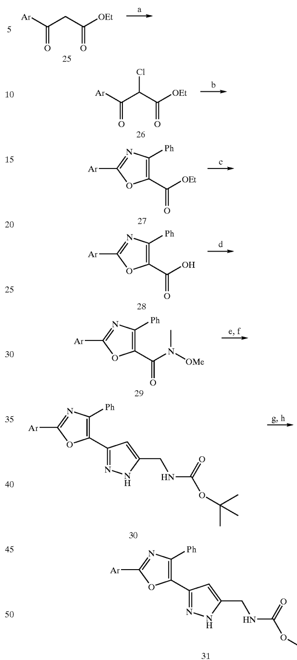
Scheme VI
