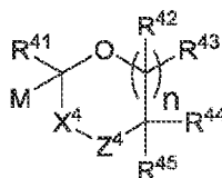
[0099] (IV)
