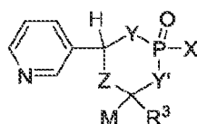
[0065] (Id)
