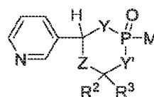
(Ie)
