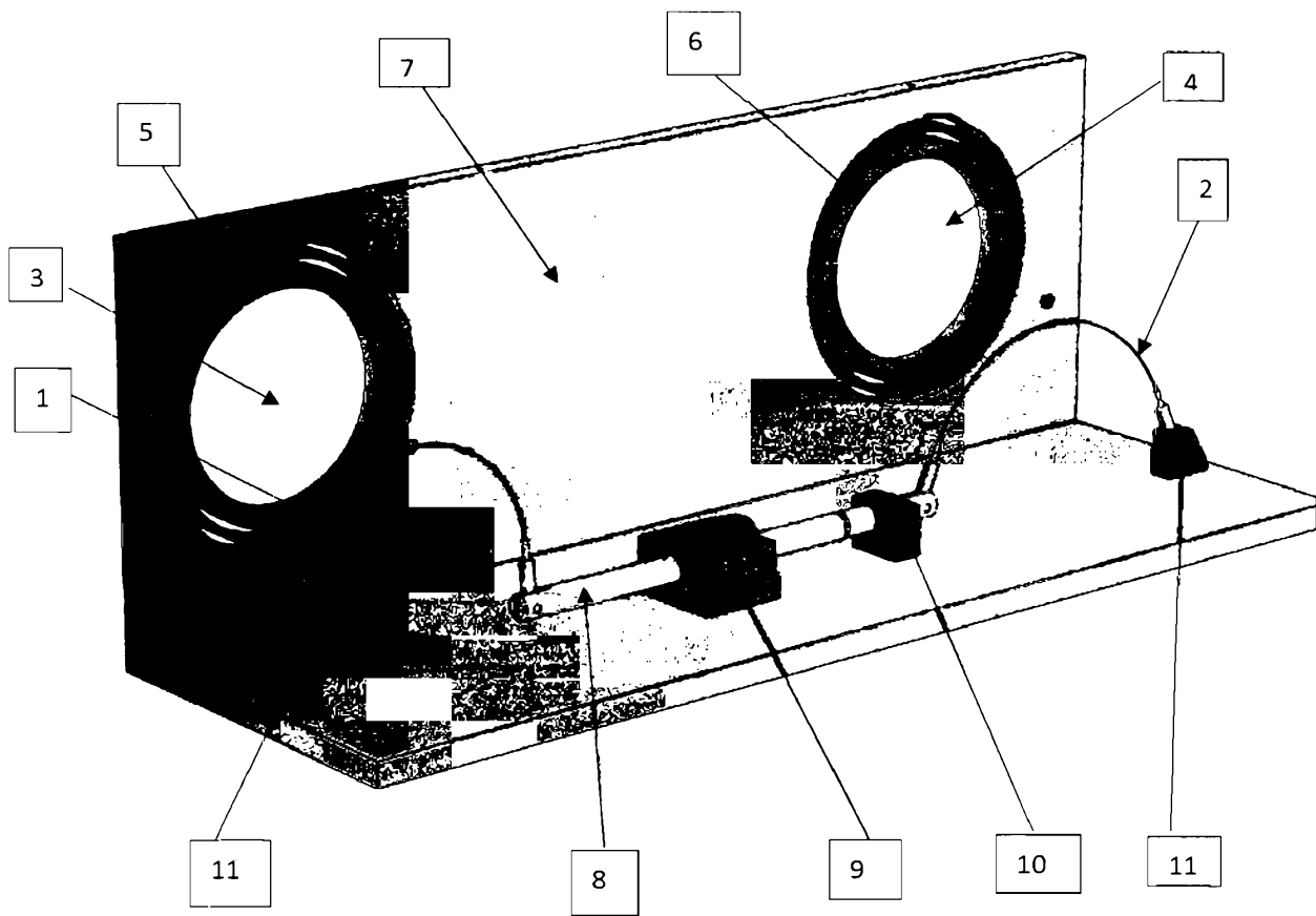
Fig. 1 Vedere de ansamblu a motorului liniar alternativ: 1,2 – elemente active din aliaj cu memoria formei; 3,4 – lentile de focalizare; 5,6 – suporturi reglabili; 7 – carcasa; 8 – ax; 9 – ghidaj; 10 – indexor; 11 – articulație
