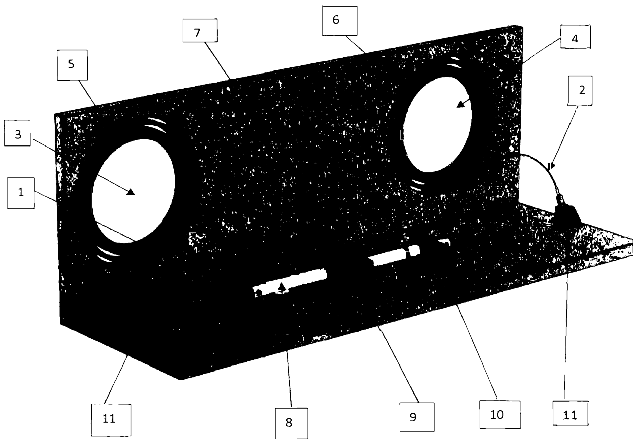
Fig. 1 - Vedere de ansamblu a motorului liniar alternativ: 1, 2 - elemente active din aliaj cu memoria formei; 3, 4 - lentile de focalizare; 5, 6 - suporturi reglabili; 7 - carcasa; 8 - ax; 9 - ghidaj; 10 - indexor; 11 - articulație
