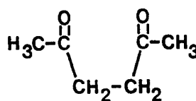
2,5-hexanedione
