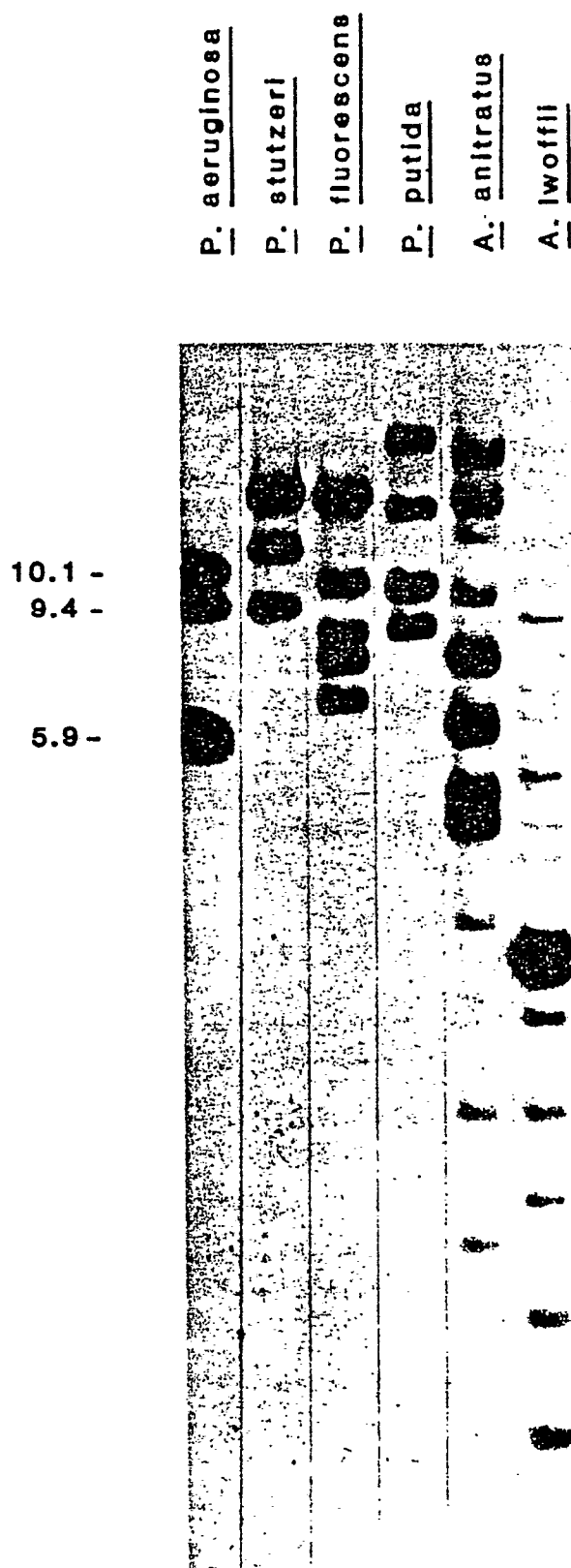
Kilobase pairs
