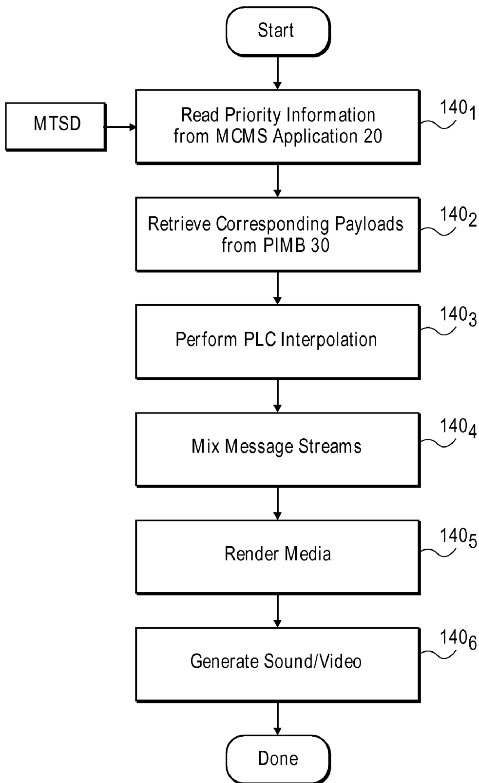
FIG. 8E
