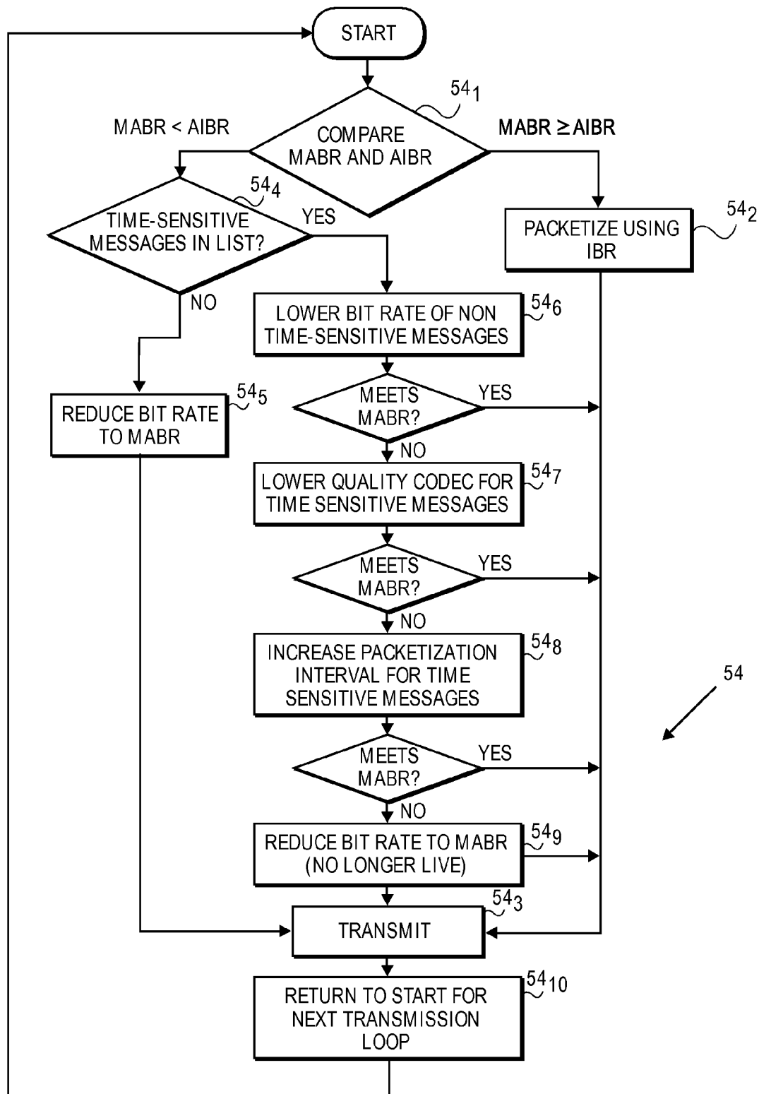
FIG. 9C
