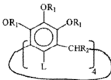
Formule I
